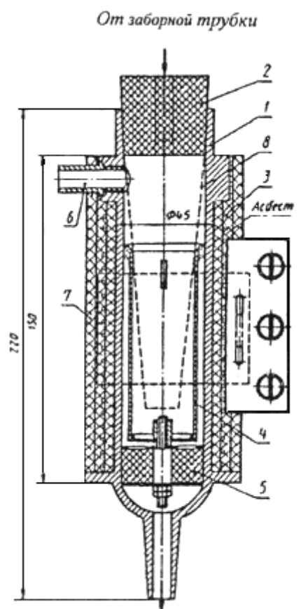
К аспирационному устройству
