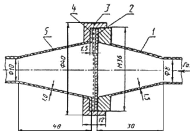
1 - диффузорный участок; 2 - мембранный фильтр; 3 - накидная гайка; 4 - опорная сетка; 5 - конфузорный участок
