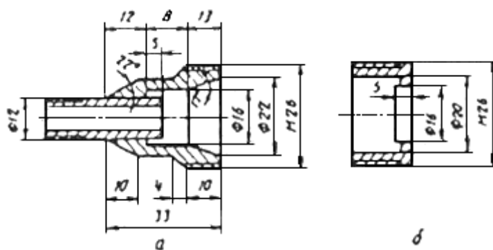
а - корпус; б - накидная гайка
