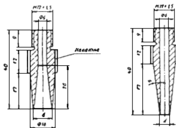
С обратным конусом
