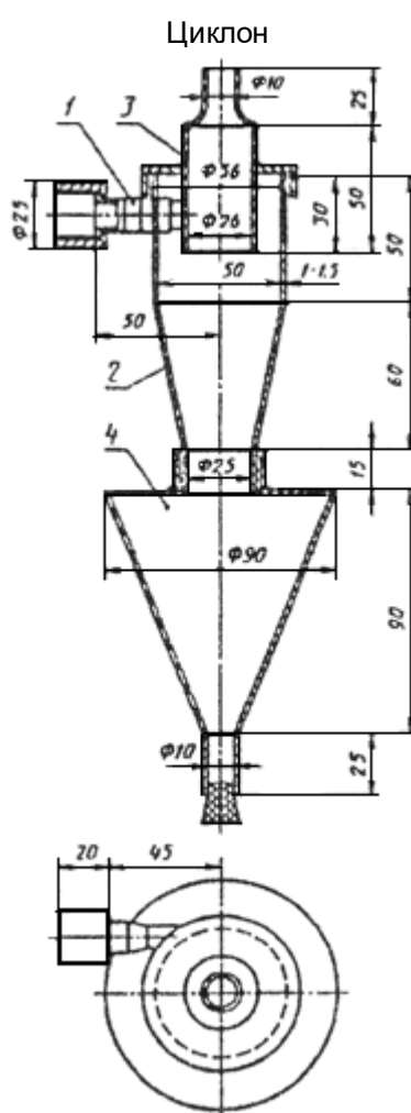
1 - входной патрубок с накидной гайкой; 2 - корпус циклона; 3 - крышка с выхлопной трубой; 4 - бункер для пыли
