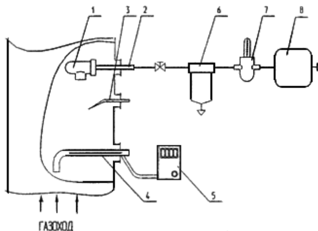
Рис.1 Схема установки для определения запыленности газа методом внутренней фильтрации 1 - патрон со стекловолокном; 2 - патронодержатель; 3 - термометр ТЦМ; 4 - напорная трубка; 5 - дифманометр ДМЦ; 6 - сброс конденсата; 7 - термометр стеклянный; 8 - аспирационное устройство
