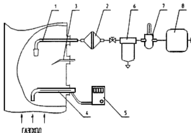
Рис.2 Схема установки для определения запыленности газа методом внешней фильтрации 1 - пылезаборная трубка; 2 - фильтродержатель АФА; 3 - термометр ТЦМ; 4 - напорная трубка; 5 - дифманометр ДМЦ; 6 - сброс конденсата; 7 - термометр стеклянный; 8 - аспирационное устройство
