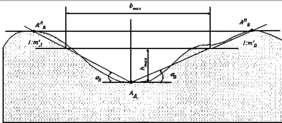
Рис.2. Поперечное сечение лога
