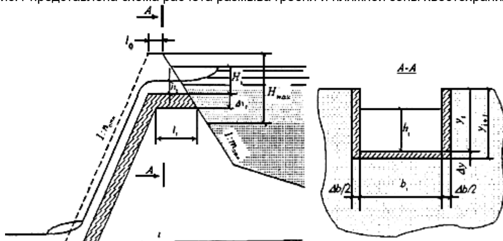
Рис.1. Схема расчета размыва прорана
