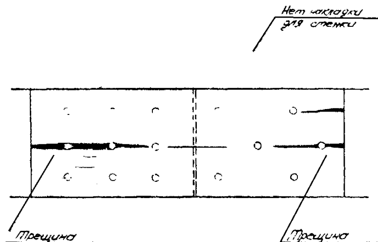
Рис. 19. Трещины в растянутом стыке нижнего пояса деревянной двутавровой балки.
