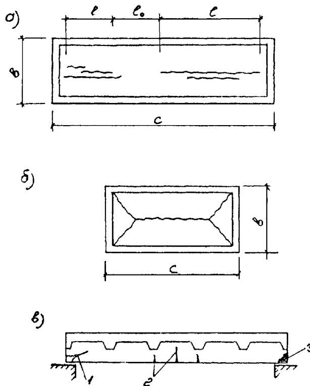
Рис. 9. Трещины при разрушении плит:
