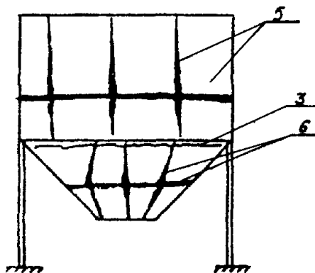
Рис. 26. Трещины от нагрузок в железобетонных бункерах:
