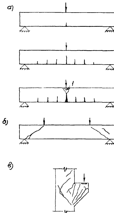
Рис. 6. Трещины при разрушении изгибаемых железобетонных элементов: а - от действия изгибающего момента на различных стадиях работы; б - от поперечной силы; в - в короткой консоле.
