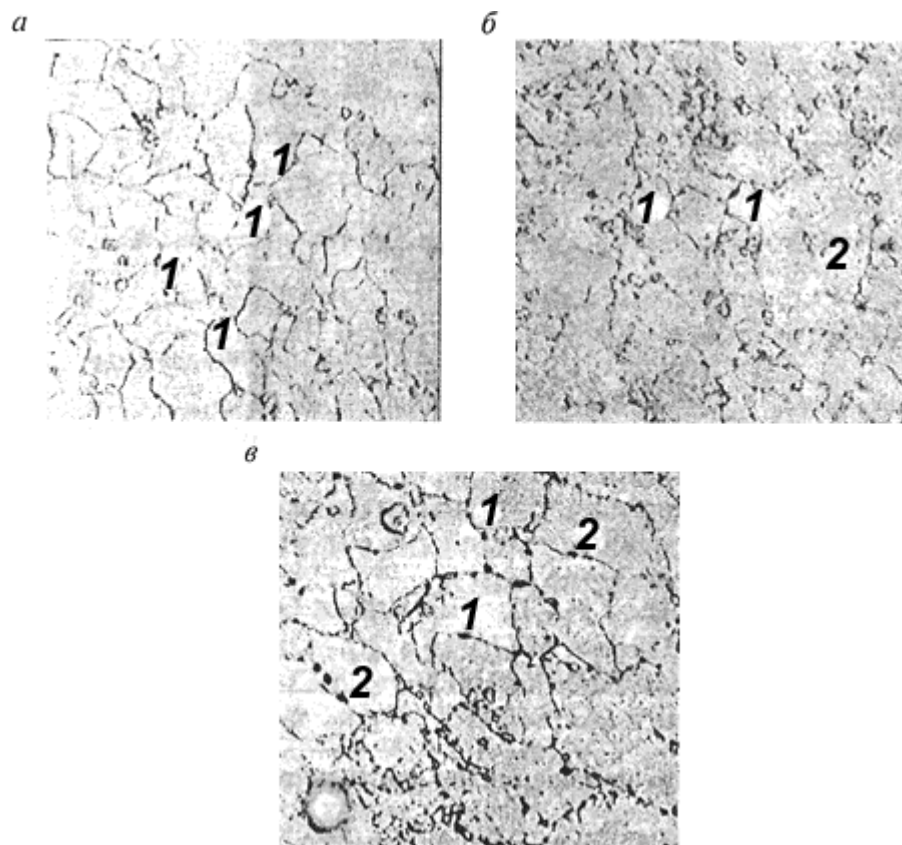
Рис.14. Микроструктура стали 12X1МФ.
