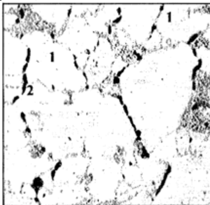
Рис.9. Микроструктура стали 12X1МФ.
