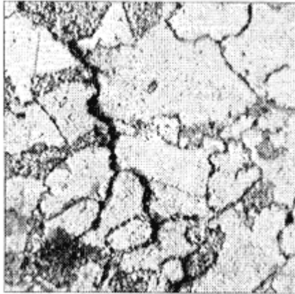
Рис.5. Микроструктура стали 12X1МФ
