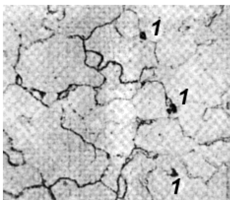
Рис.15. Микроструктура стали 12X1МФ.
