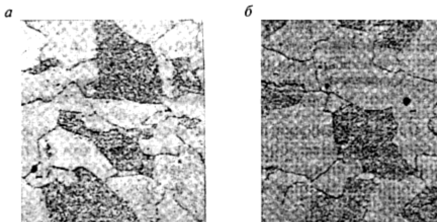
Рис.10. Микроструктура стали 12X1МФ.
