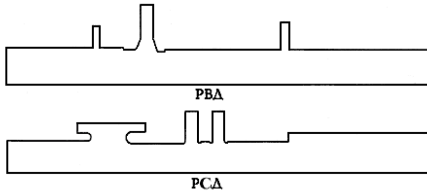
Рис.2. Расчетные схемы роторов для определения напряжений методом граничных интегральных уравнений
