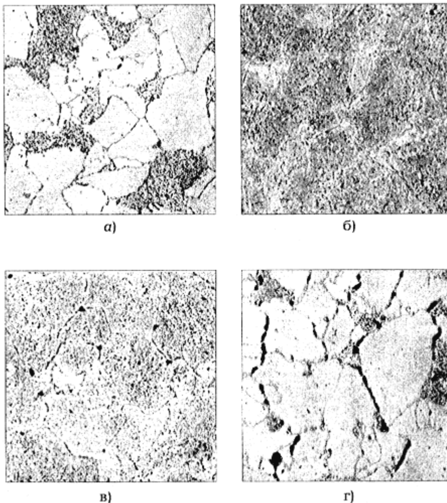
Рис.4. Микроструктура сталей 12X1MФ (а, г) и 15X1M1Ф (б, в)
