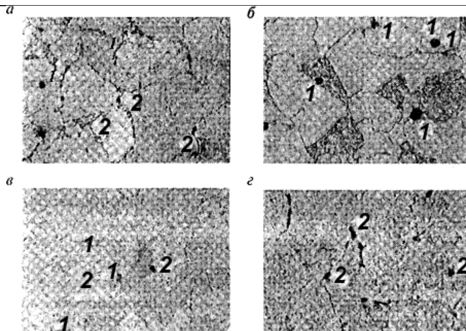
Рис.11. Микроструктура сталей 12X1MФ (а, б) и 15X1M1Ф (в, г).
