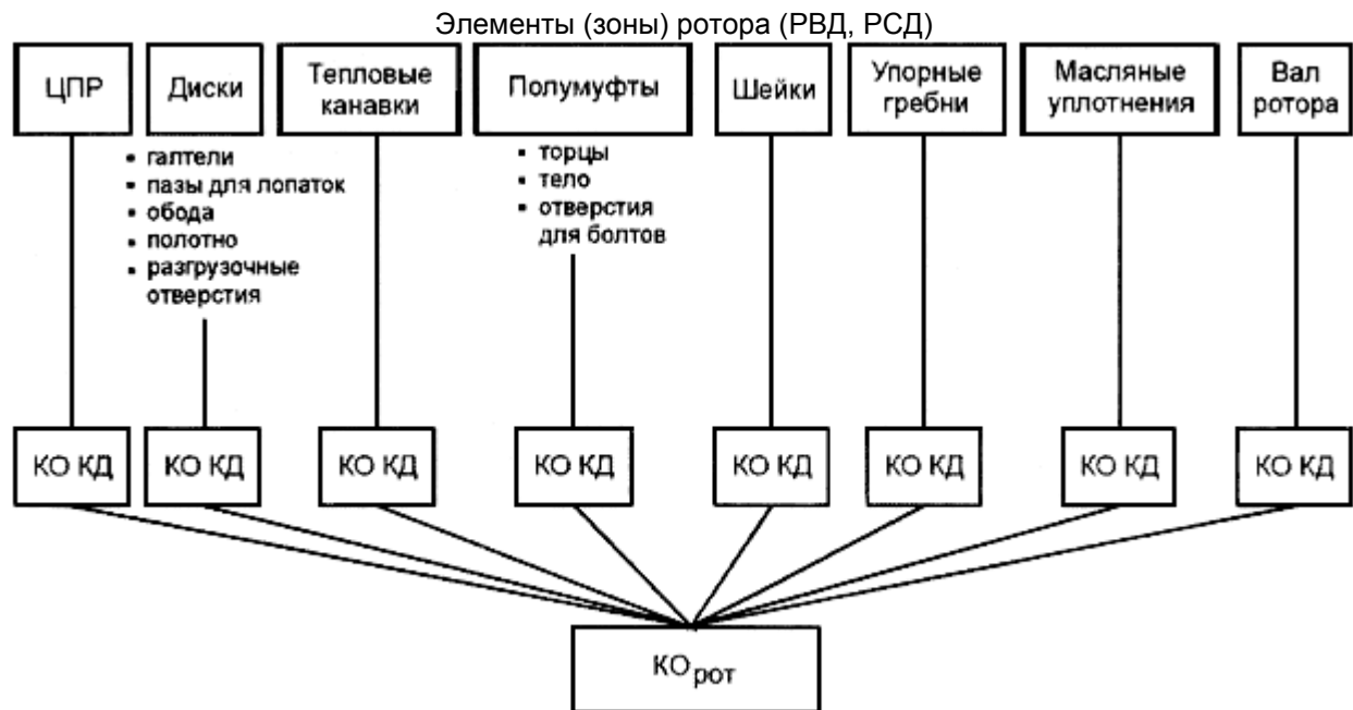
Рис.3. Блок-схема экспертизы состояния ротора
