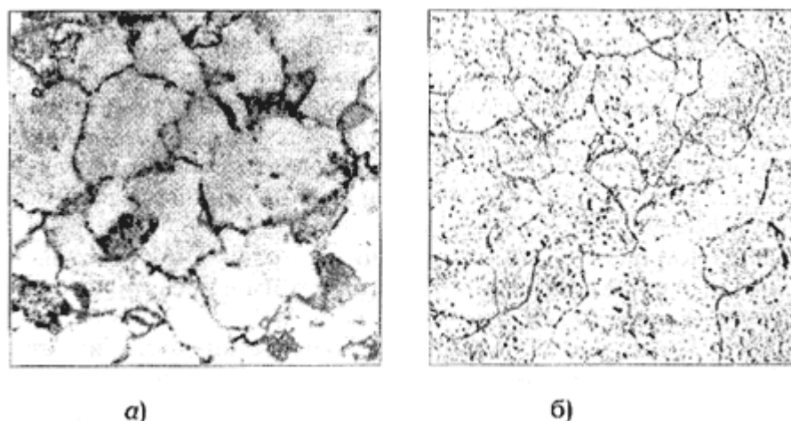
Рис.8 Микроструктура сталей 12X1МФ (а) и 15X1М1Ф (б).
