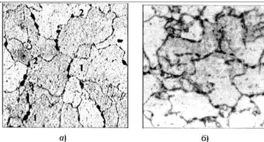
Рис.7. Микроструктура стали 12X1МФ
