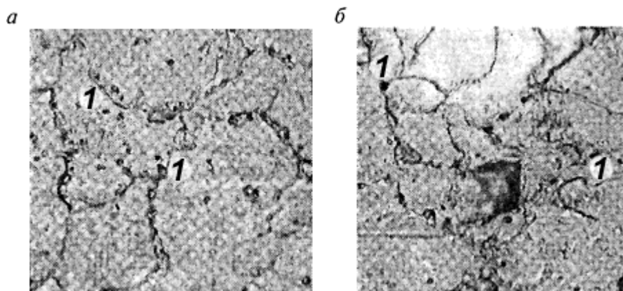
Рис.13. Микроструктура стали 12Х1МФ.
