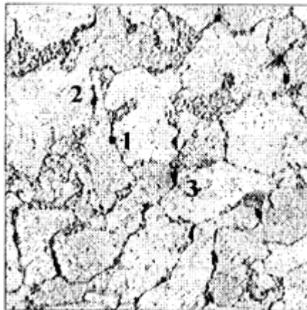
Рис.6. Микроструктура стали 12X1МФ
