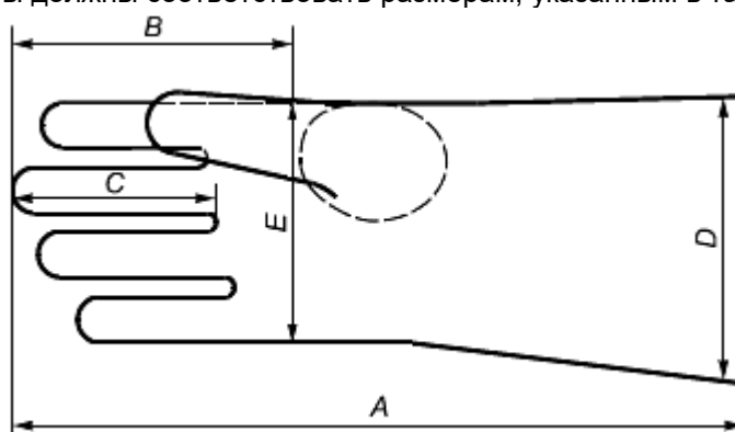
Рисунок 1 - Внутренние размеры ЗАЩИТНЫХ ПЕРЧАТОК
