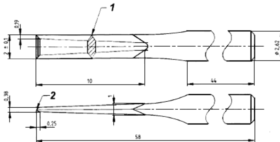
1 - острый прямоугольный край с обеих сторон лезвия, сужающийся на конус к точке; 2 - острие лезвия
