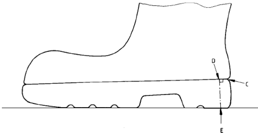
Рисунок A.1 - Измерение толщины каблука
