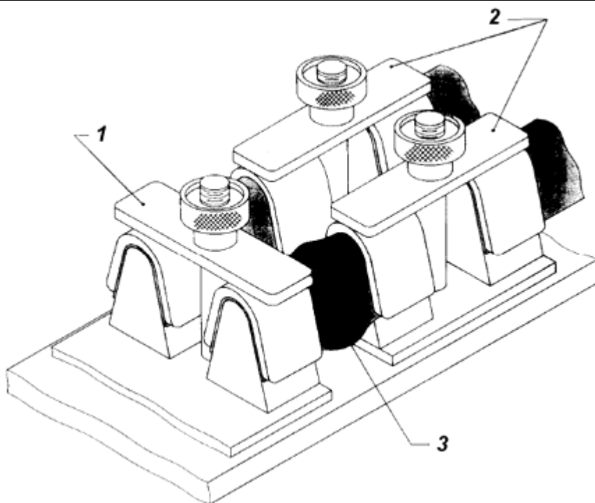
1 - неподвижный зажим; 2 - подвижный зажим; 3 - образец для испытаний
