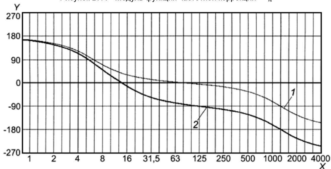
Рисунок В.11 - Модуль функции частотной коррекции W_h
