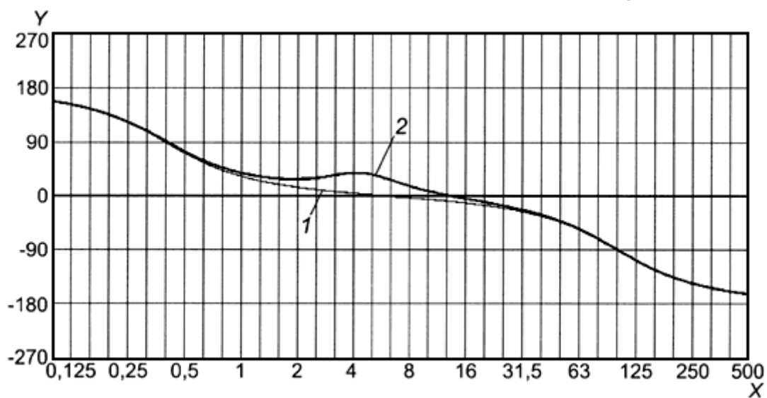
Рисунок В.13 - Модуль функции частотной коррекции W_j
