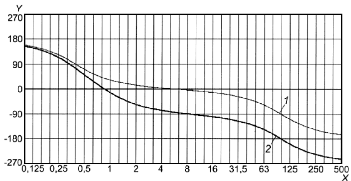
Рисунок В.7 - Модуль функции частотной коррекции W_e
