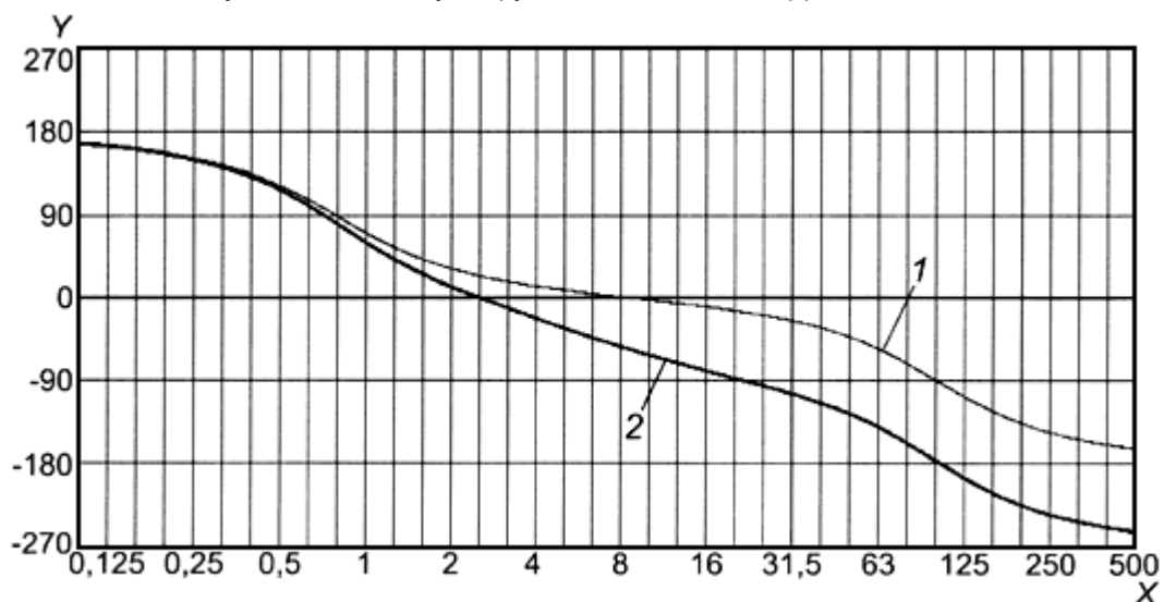
Рисунок В.17 - Модуль функции частотной коррекции W_m
