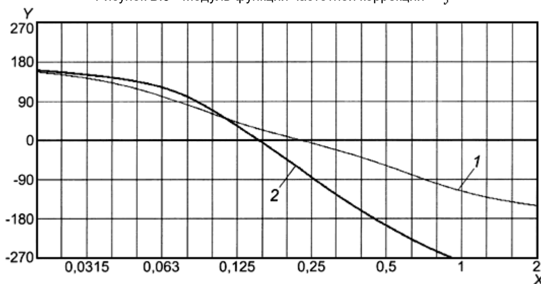
Рисунок В.9 - Модуль функции частотной коррекции W_f
