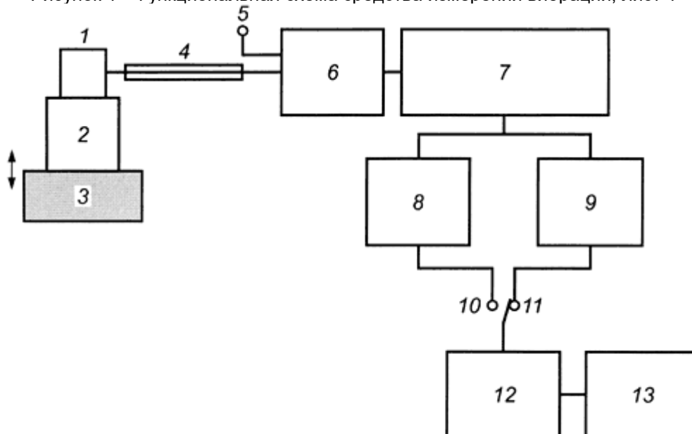
а) Функциональная схема для преобразования сигнала во временной области Рисунок 1 - Функциональная схема средства измерений вибрации, лист 1
