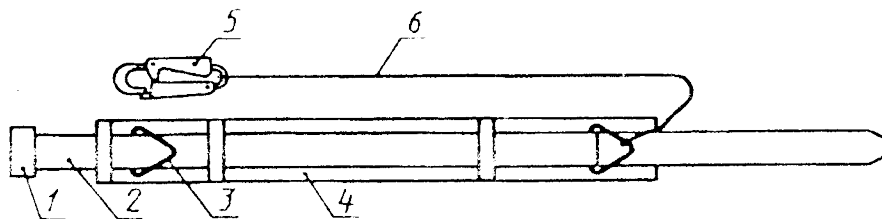
Рисунок 1 - Безлямочный пояс, тип А
