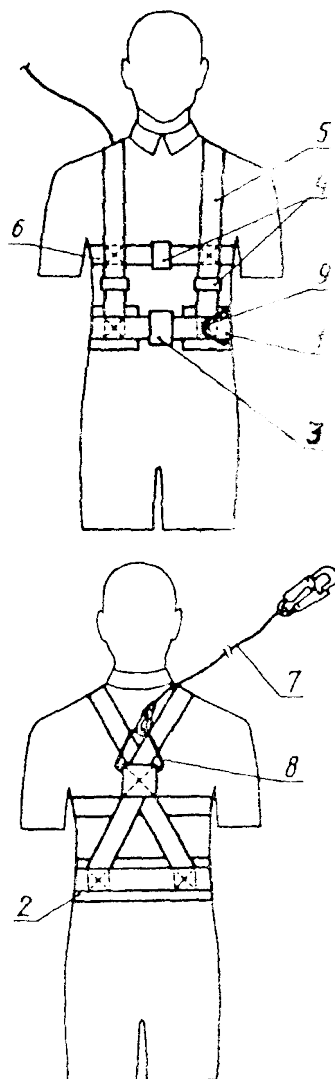
Рисунок 3 - Лямочный пояс, тип В
