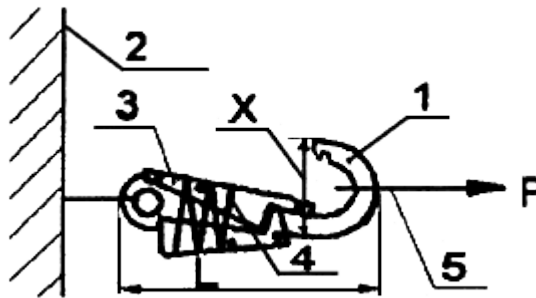
Рисунок 8а - Схема испытания карабина статической нагрузкой
