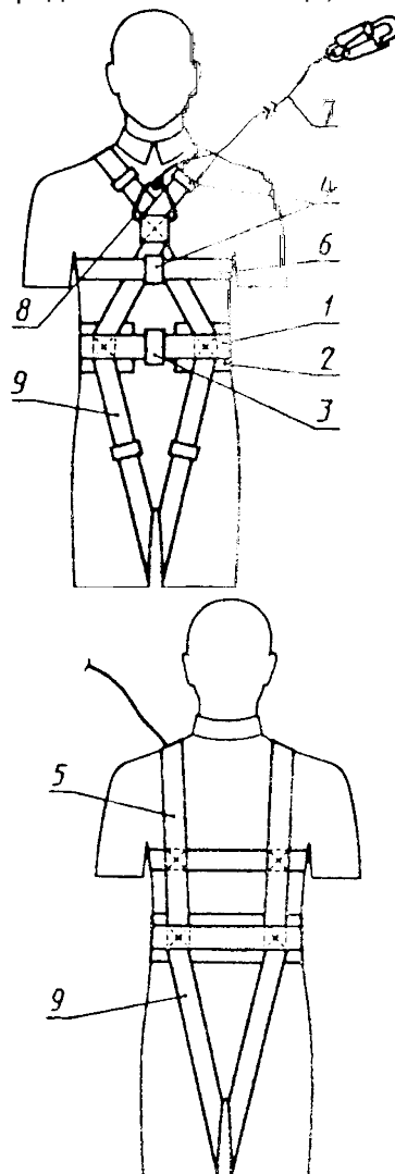
Рисунок 6 - Лямочный пояс, тип Е
