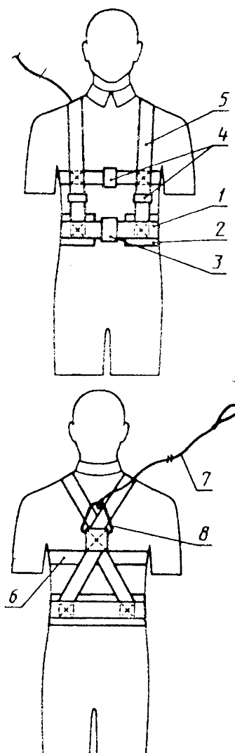
Рисунок 4 - Лямочный пояс, тип Г
